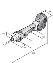
AGSZ 18-280 BL
