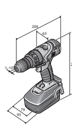
ASB 18 Q
