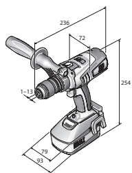
ASCM 18 QM
