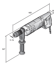
BOS 16-2
