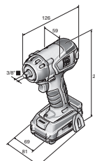
ASCD 12-150 W8C
