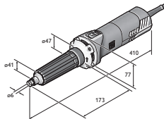
GSZ 8-280 PEL
