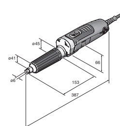
GSZ 4-90 EL
