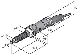
GSZ 11-320 PERL
