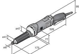
GSZ 11-90 PERL
