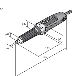
GSZ 4-280 EL
