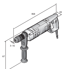
BOS 16
