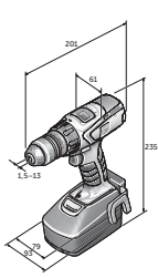
ASCM 18 QSW
